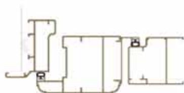
PROFILO ANTA RUSTICA CON TELAIO A IMBOTTE
